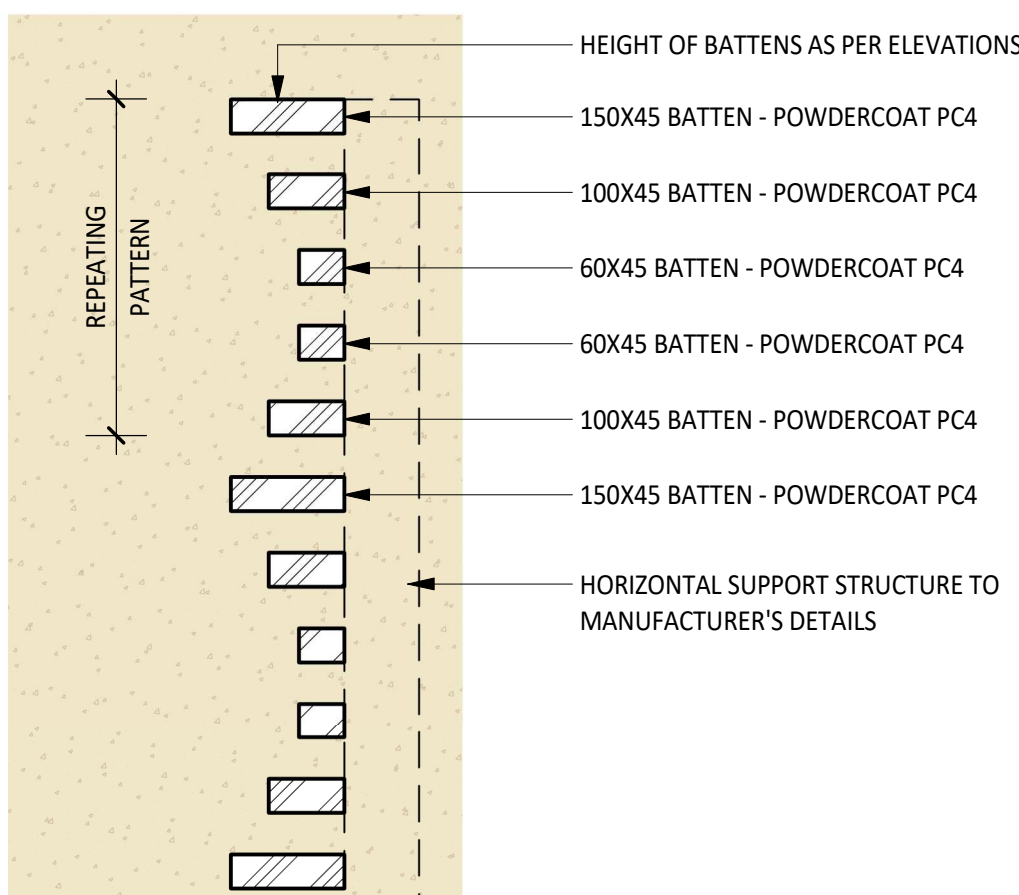
2 PLAN DETAIL - BATTEN SCREEN TYPE 1 - BST 1 21-01 1 : 10
